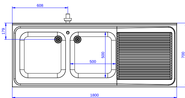
Felülnézet
